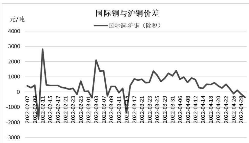
图 1 国际铜与沪铜价差
